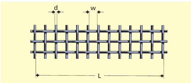
Bild 3: Messreihe mit bestimmter Länge, für Maschenweiten 1 mm bis 16 mm.
