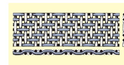
Drahtgewebe, Körperbindung
